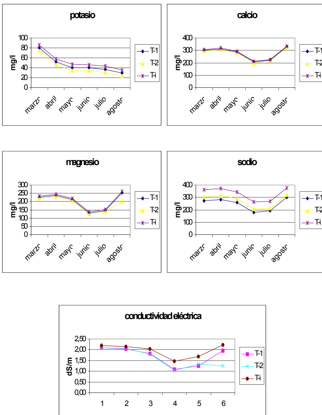
Figura 1: Evolución mensual de cationes y conductividad eléctrica en la solución del suelo.
